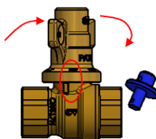
4. Girar el accionamiento hasta la posición de bloqueo deseada (bloqueo 10% apertura). / Rotate the handle until the required locked position (Lock in 10% opening).
