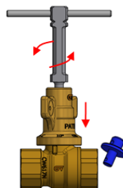
5. Introducir de nuevo la llave especial hasta enganchar el tornillo y girar en sentido anti-horario. El accionamiento quedará bloqueado y no se podrá girar. / Fit the special key again, engage the screw and rotate counter-clockwise. The handle will remain locked and you can not rotate it.
